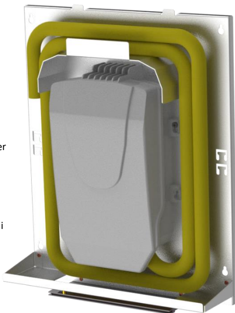
1 Bagplade monteres på væg
